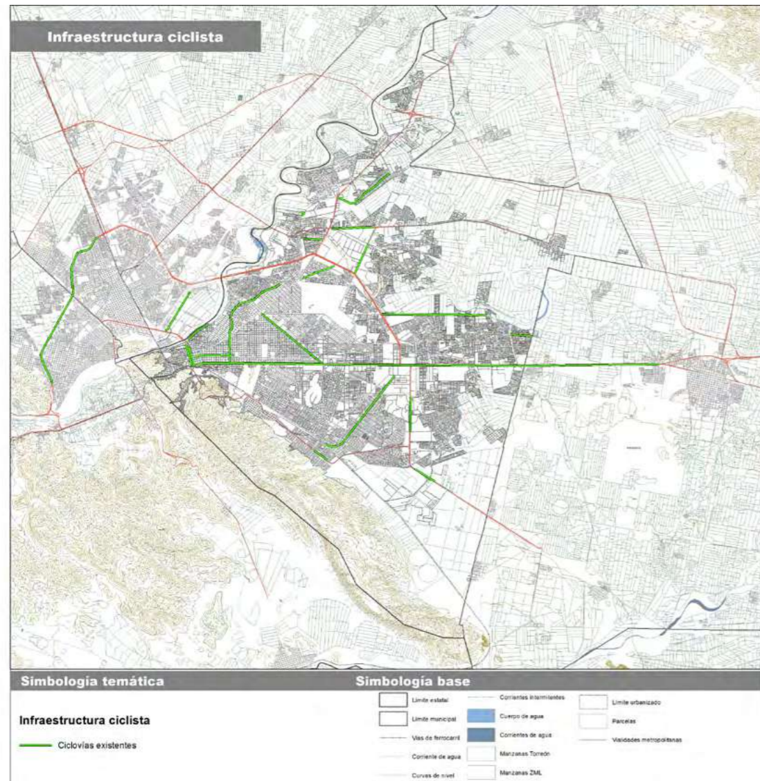
Mapa 10. Infraestructura ciclista.
